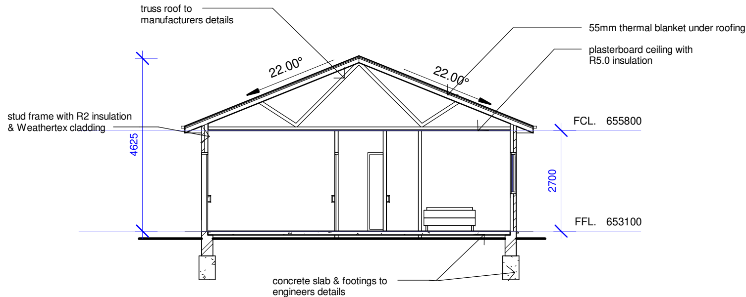
1 SECTION A 1 : 100
