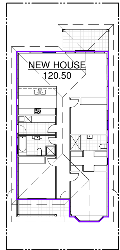
2 AREAS-01 1 : 200
